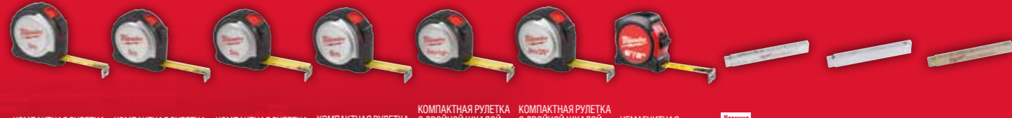
КОМПАКТНАЯ РУЛЕТКА С МЕТРИЧЕСКОЙ ШКАЛОЙ (3 М, ШИРИНА ЛЕНТЫ – 16 ММ) 4932451637 КОМПАКТНАЯ РУЛЕТКА С МЕТРИЧЕСКОЙ ШКАЛОЙ (5 М, ШИРИНА ЛЕНТЫ – 19 ММ) 4932451638 КОМПАКТНАЯ РУЛЕТКА С МЕТРИЧЕСКОЙ ШКАЛОЙ (5 М, ШИРИНА ЛЕНТЫ – 25 ММ) 4932451639 КОМПАКТНАЯ РУЛЕТКА С МЕТРИЧЕСКОЙ ШКАЛОЙ (8 М, ШИРИНА ЛЕНТЫ – 25 ММ) 4932451640 КОМПАКТНАЯ РУЛЕТКА С ДВОЙНОЙ ШКАЛОЙ (5 М/16 ФУТОВ, ШИРИНА ЛЕНТЫ – 25 ММ) 4932451641 КОМПАКТНАЯ РУЛЕТКА С ДВОЙНОЙ ШКАЛОЙ (8 М/26 ФУТОВ, ШИРИНА ЛЕНТЫ – 25 ММ) 4932451642 НЕМАГНИТНАЯ РУЛЕТКА С ДВОЙНОЙ ШКАЛОЙ (2 М/6 ФУТОВ) 48225502 Новинка СКЛАДНОЙ МЕТР ИЗ КОМПОЗИТНОГО МАТЕРИАЛА 4932459301 Новинка ДЕРЕВЯННЫЙ СКЛАДНОЙ МЕТР 4932459302 Новинка УЗКИЙ ДЕРЕВЯННЫЙ СКЛАДНОЙ МЕТР 4932459303
